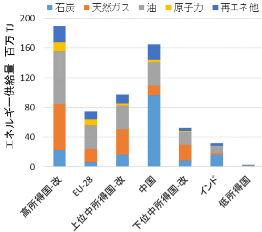
図-28 グループ別 一次エネルギー供給量 (2020年) 出所: 米国eia、Internationalデータ
