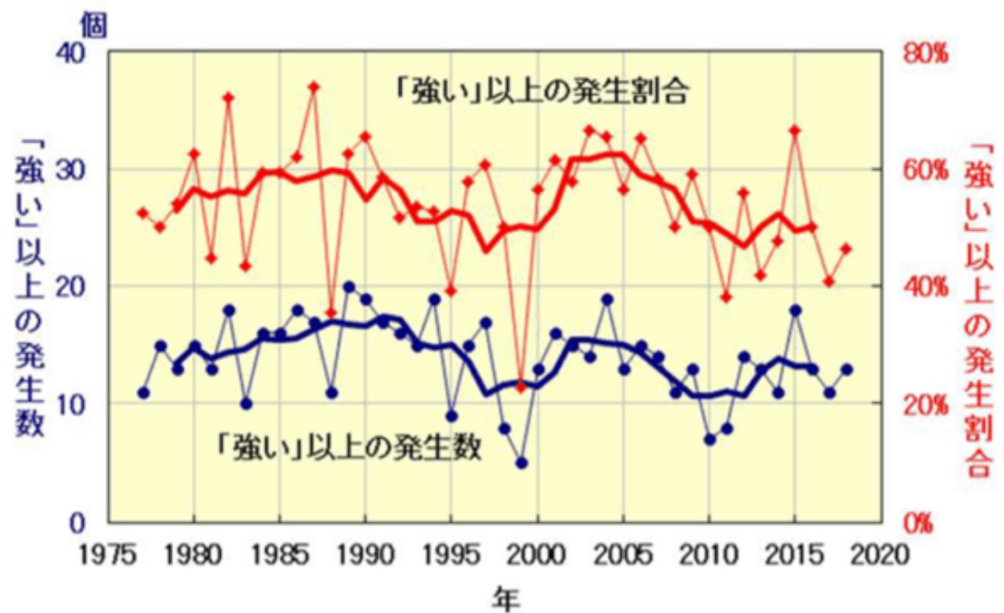
図 2.4-3 「強い」以上の勢力となった台風の発生数と全発生数に対する割合の経年変化 細い実線は、「強い」以上の勢力となった台風の発生数（青）と全台風に対する割合（赤）の経年変化。太い実線は、それぞれの5年移動平均。
