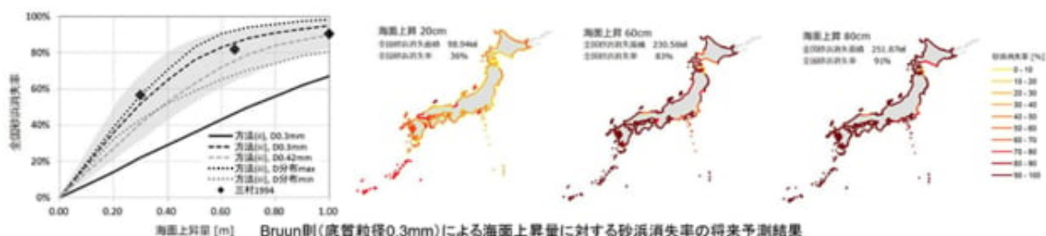
Brunn則(底質粒径0.3mm)による海面上昇量に対する砂浜消失率の将来予測結果
