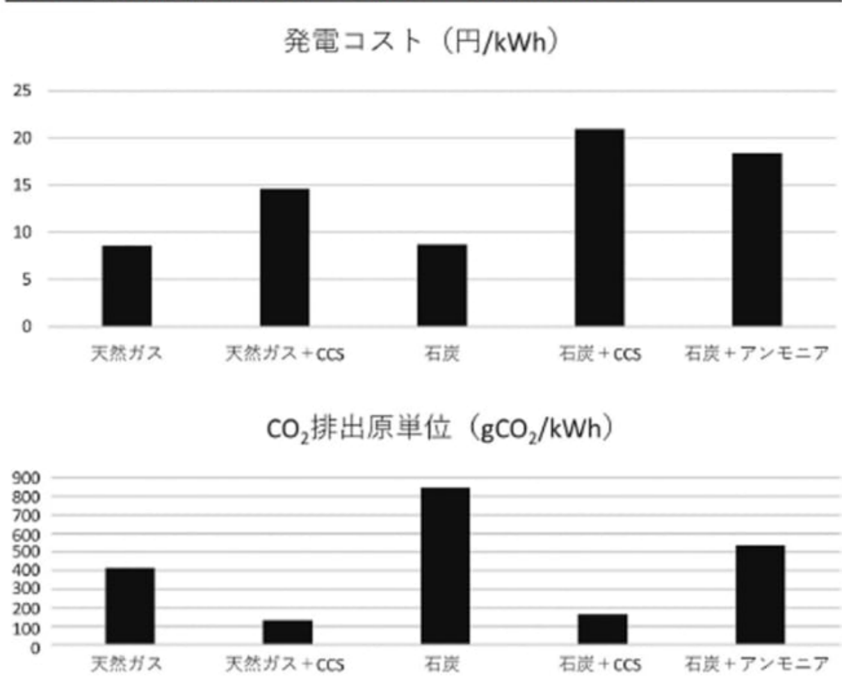
図表 37 化石燃料由来の発電コスト及び CO 2 排出原単位の試算
